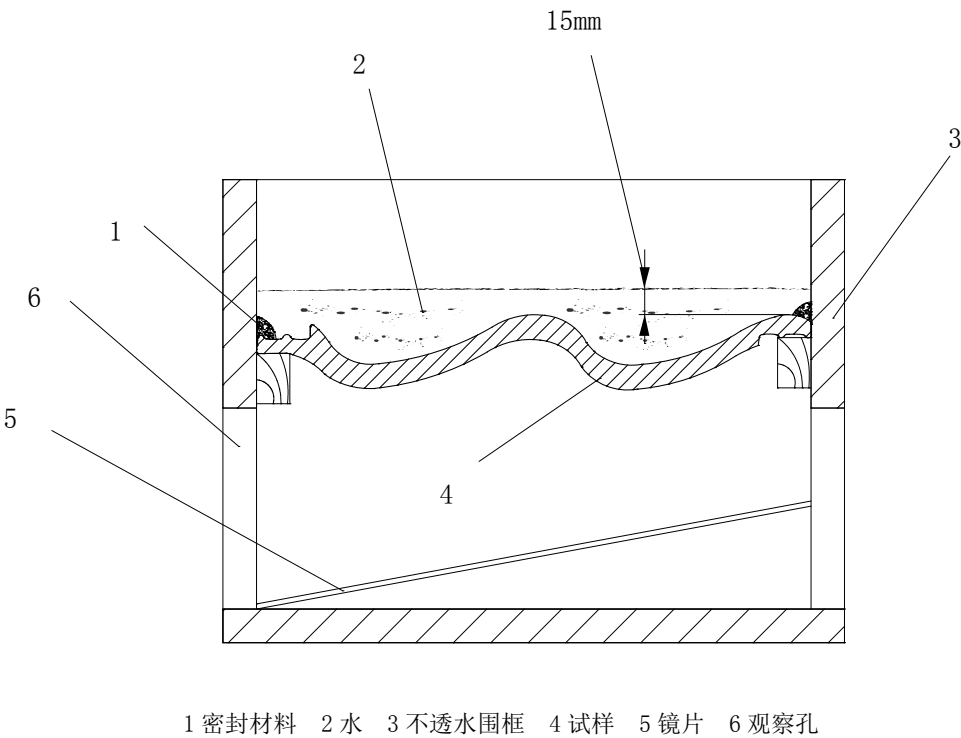
图 D1 抗渗试验装置示意
