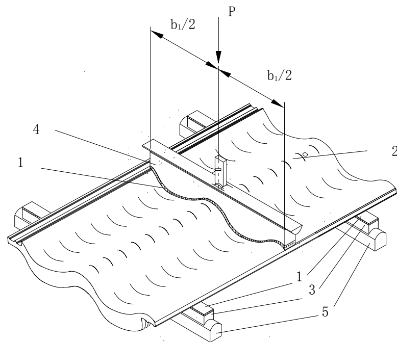
1 弹性垫层 2 试样 3 硬质木条 4 平衡物 5 支座
