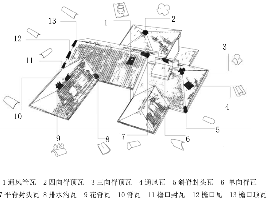
图 3 配件瓦结构形状及名称
