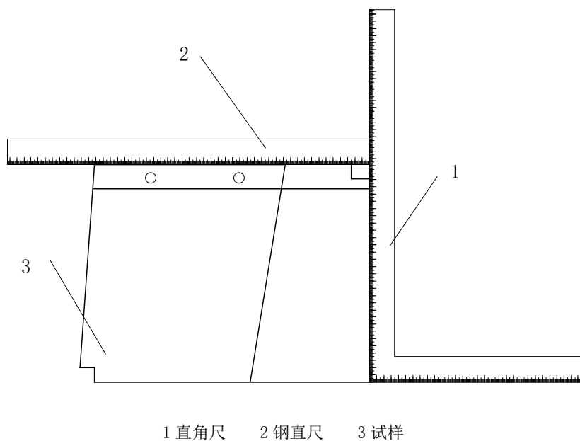
图 A1 瓦角为非直角形状时边长的测量示意
