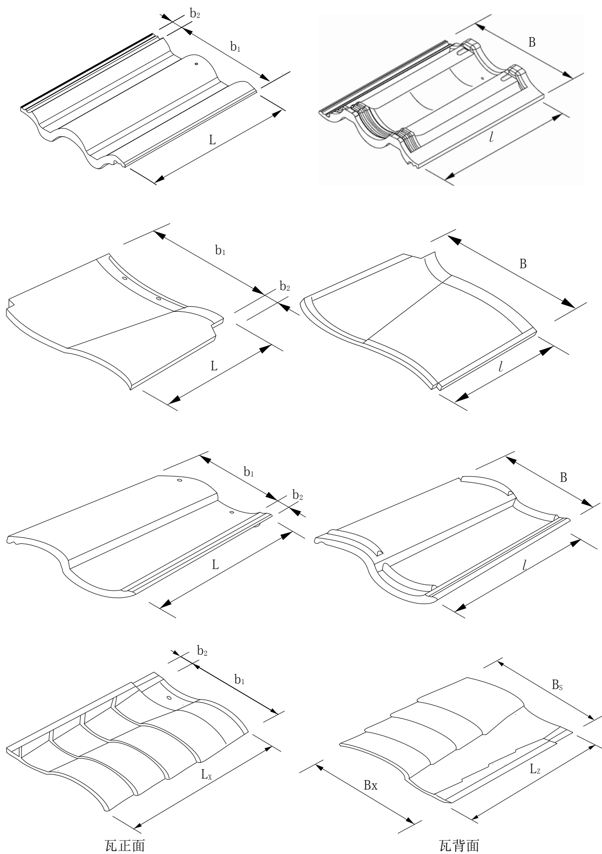
图1 波形瓦结构形状
