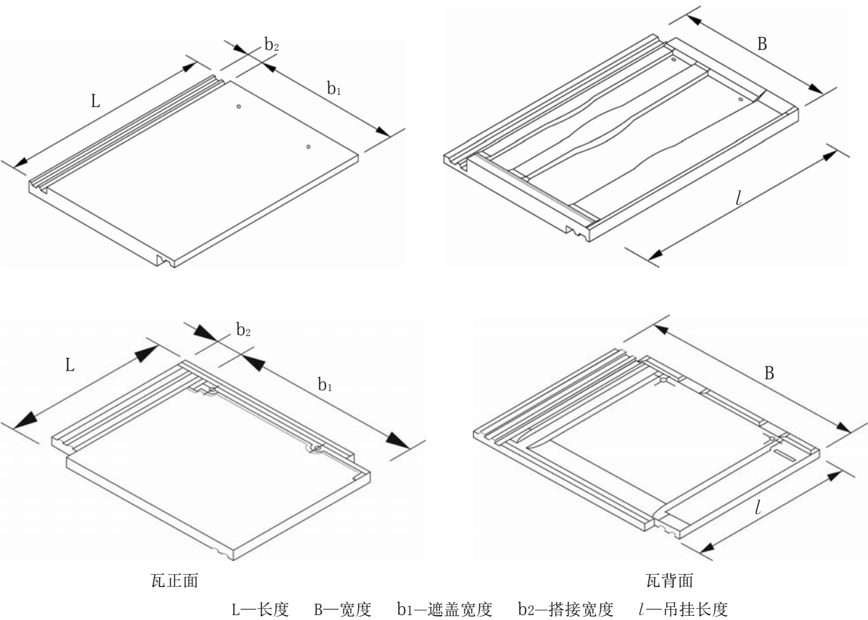
图 2 平板瓦结构形状
